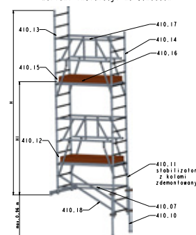
RA 330 R-R Wariant instalacji na schodach
